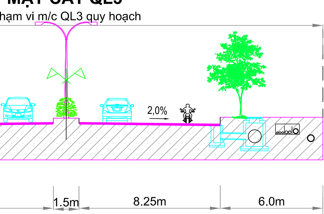
MẶT CẮT QL3
