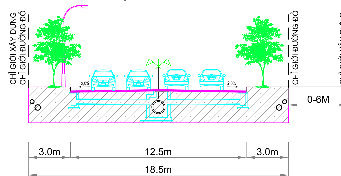
MẶT CẮT 1 - 1
