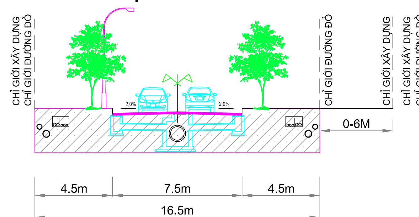
MẶT CẮT 4 - 4
