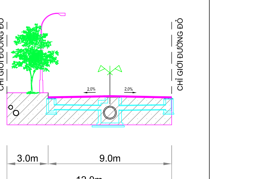
MẶT CẮT QL3
