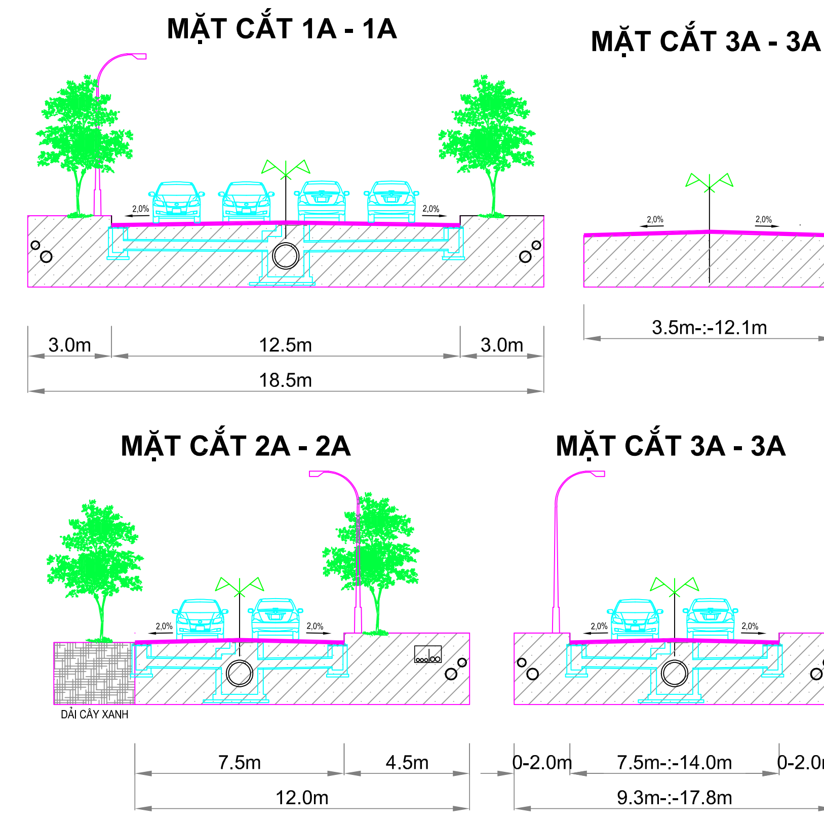
MẶT CẮT ĐẠI DIỆN GIAO THÔNG NỘI BỘ KHU NHÀ Ở XH
